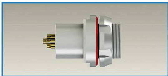
真封型插座
