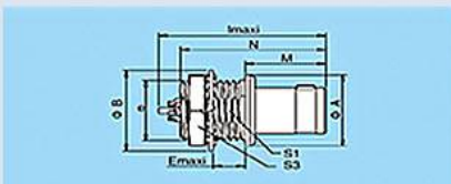
固定式插头
