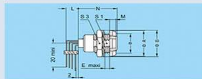
双螺母固定式插座
