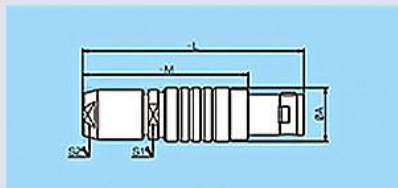
直式插头
