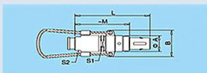
直式带拉绳插头
