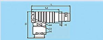
90°弯角式插头
