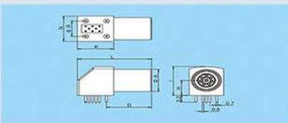
插座【焊接或螺母固定】
