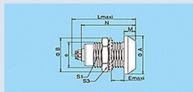
固定式插座
