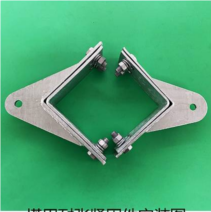
塔用耐张紧固件安装图
