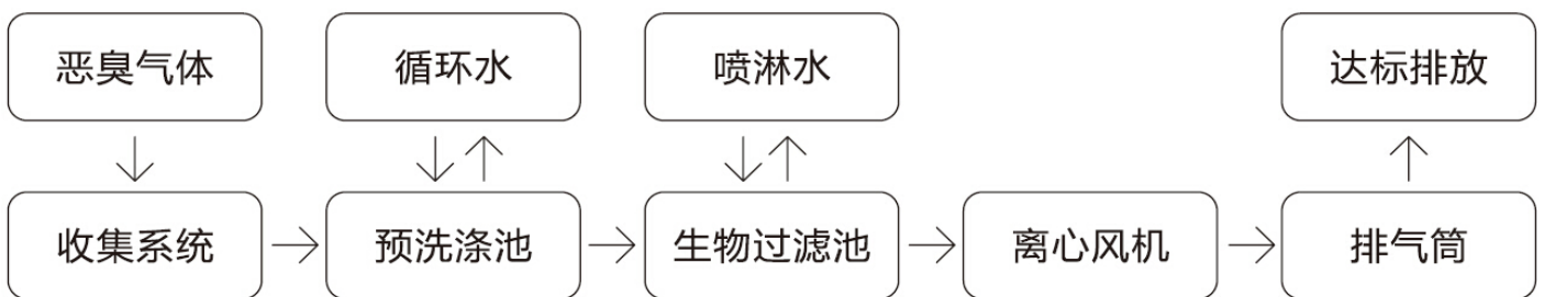
生物除臭流程图
