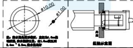
结构装配图
