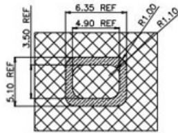
面板开孔参考尺寸
