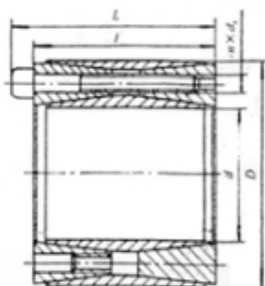
Z18 型胀紧联接套的基本尺寸
