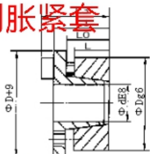
Z8型胀紧联接套的基本尺寸
