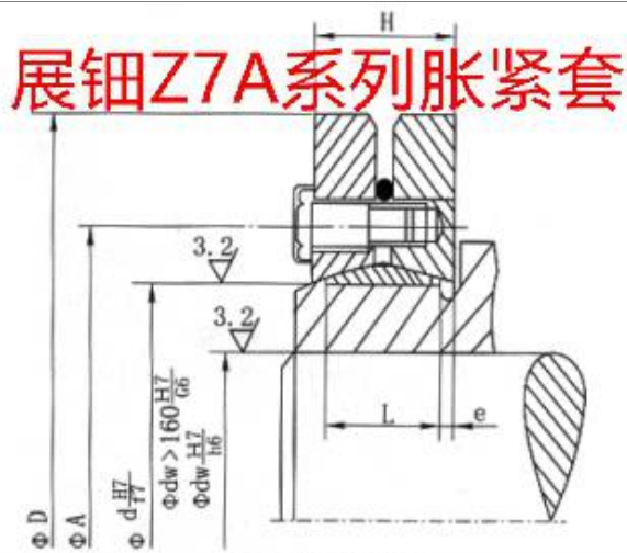
Z7A型胀紧套的基本尺寸
