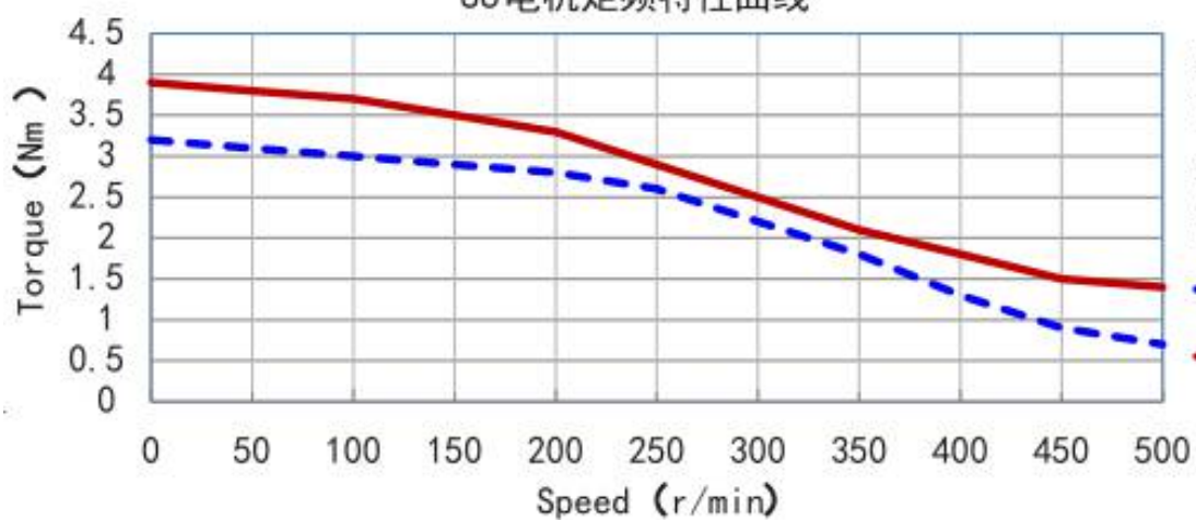
86电机矩频特性曲线
