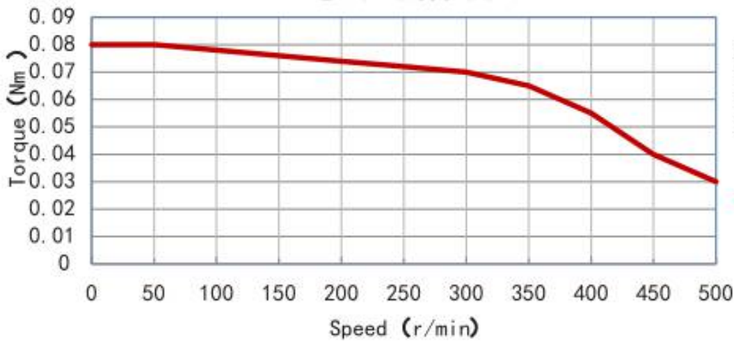
28电机矩频特性曲线
